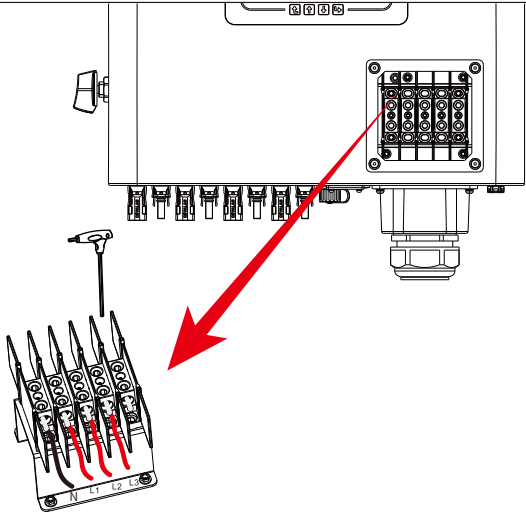
Imagen 5.7 Conexión de entrada de CA
