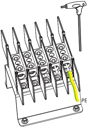
Imagen 5.8 La instalación del cable de tierra de la carcasa
