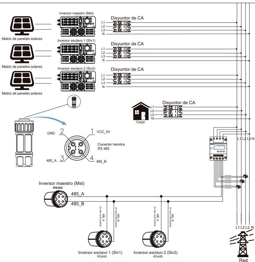
Imagen 7.31 Diagrama de conexión CHINT (tabla de paso)
