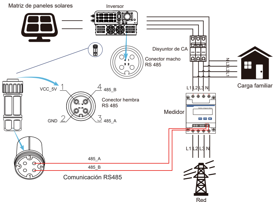
Imagen 7.10 Diagrama de conexión del medidor CHINT
