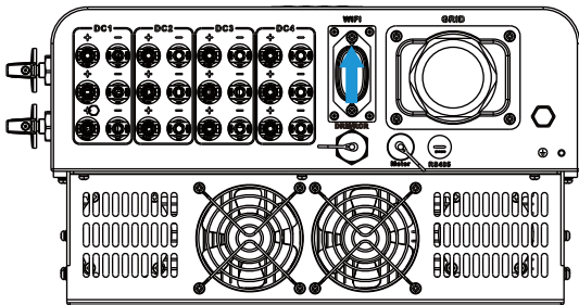
Imagen 5.10 Diagrama de instalación del registrador de datos
