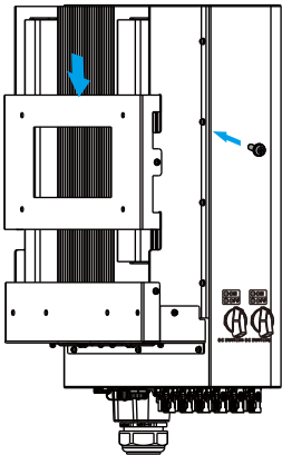
Imagen 4.6 Instalación del inversor
