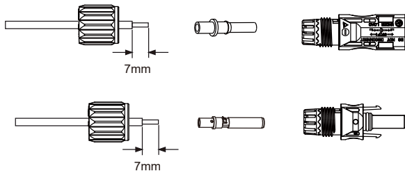
Imagen 5.3 Desmonte la tuerca ciega del conector
