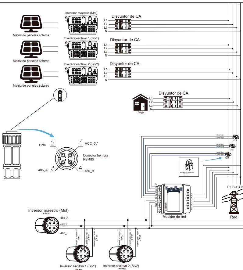
Imagen 7.23 Diagrama de conexión (electricidad trifásica)
