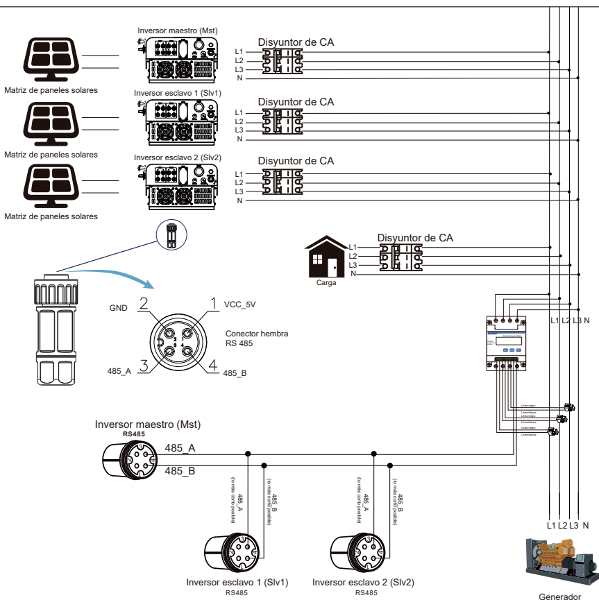
Imagen 7.33 Diagrama de conexión CHINT (tabla de paso)
