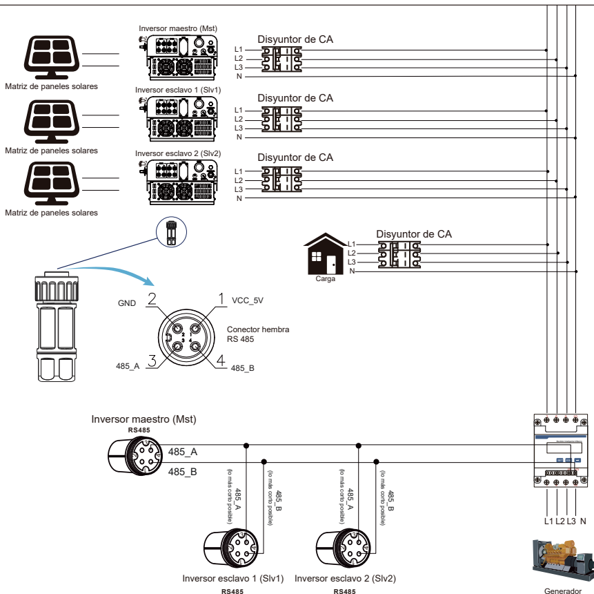
Imagen 7.29 Diagrama de conexión CHINT (tabla de paso)
