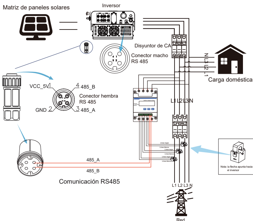
Imagen 7.14 Diagrama de conexión del medidor CHINT
