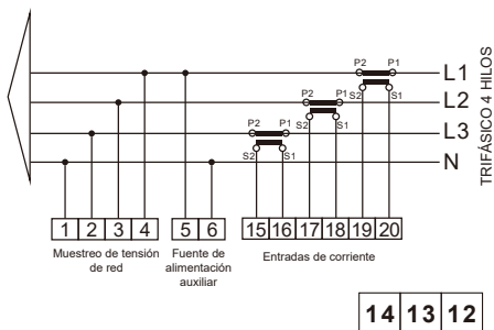
Imagen 7.22 Medidor Eastron
