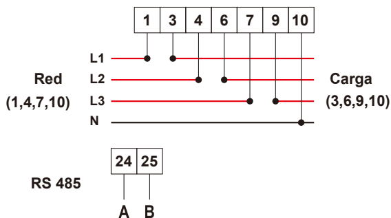
Imagen 7.9 Medidor CHINT
