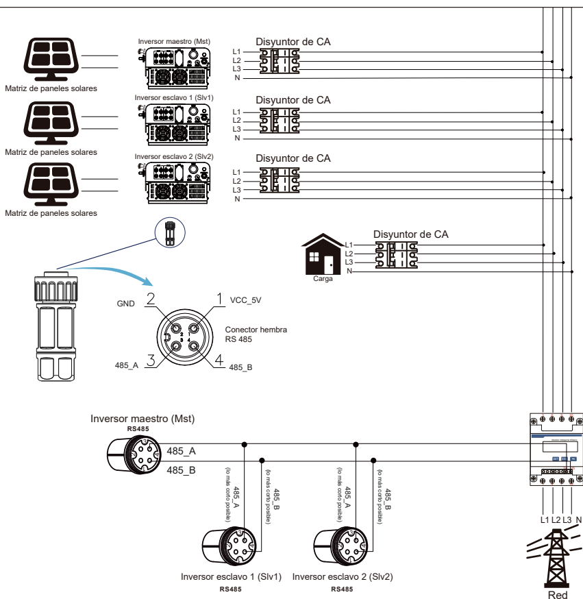
Imagen 7.27 Diagrama de conexión CHINT (tabla de paso)
