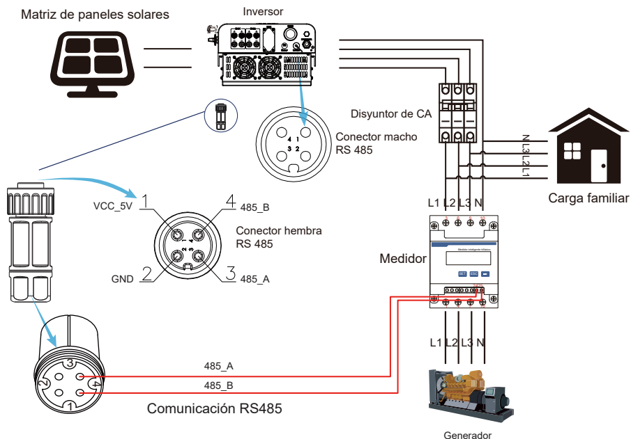
Imagen 7.12 Diagrama de conexión del medidor CHINT
