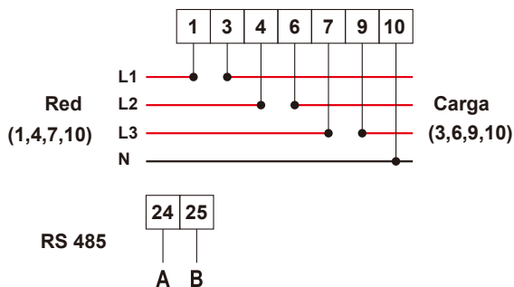
Imagen 7.11 Medidor CHINT
