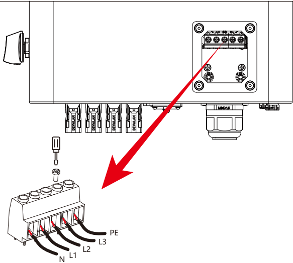
Imagen 5.7 Conexión de entrada de CA
