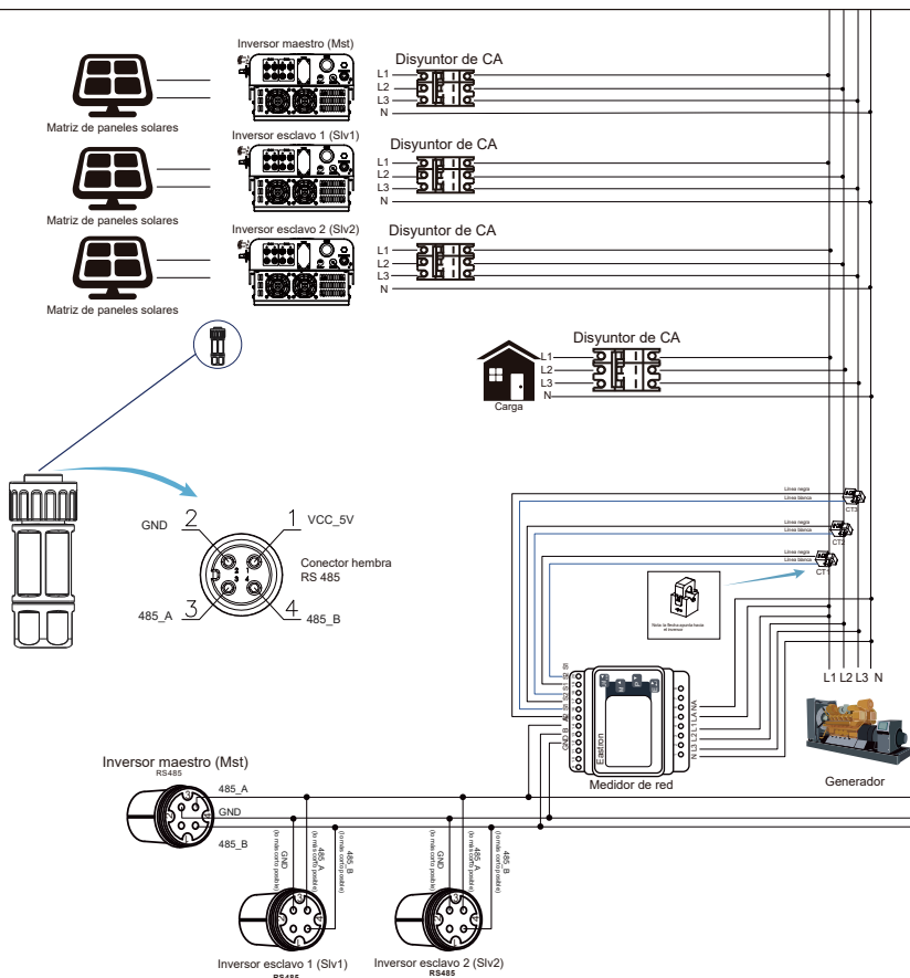
Imagen 7.25 Diagrama de conexión (electricidad trifásica)
