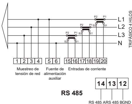
Imagen 7.7 Medidor Eastron
