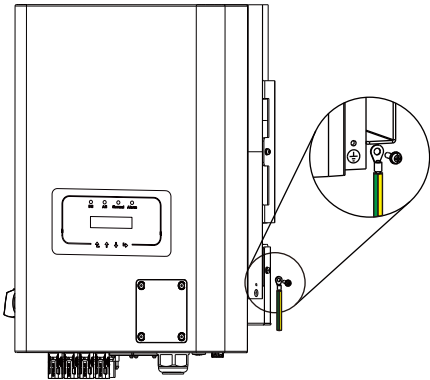
Imagen 5.8 La instalación del cable de tierra de la carcasa
