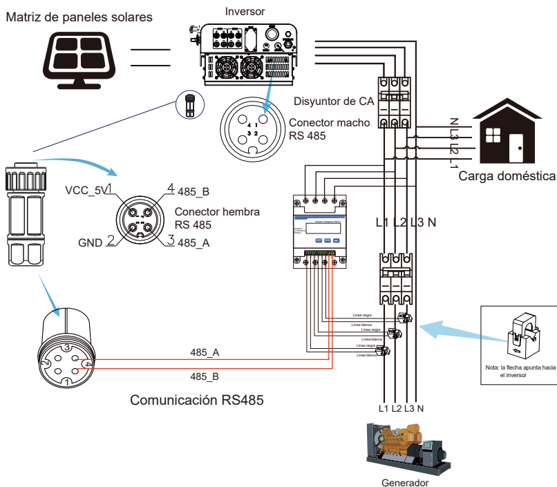
Imagen 7.16 Diagrama de conexión del medidor CHINT
