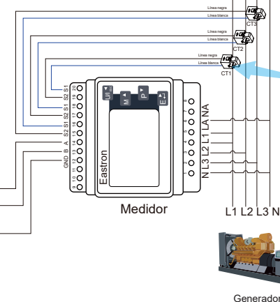
Imagen 7.8 Diagrama de conexión del medidor Eastron
